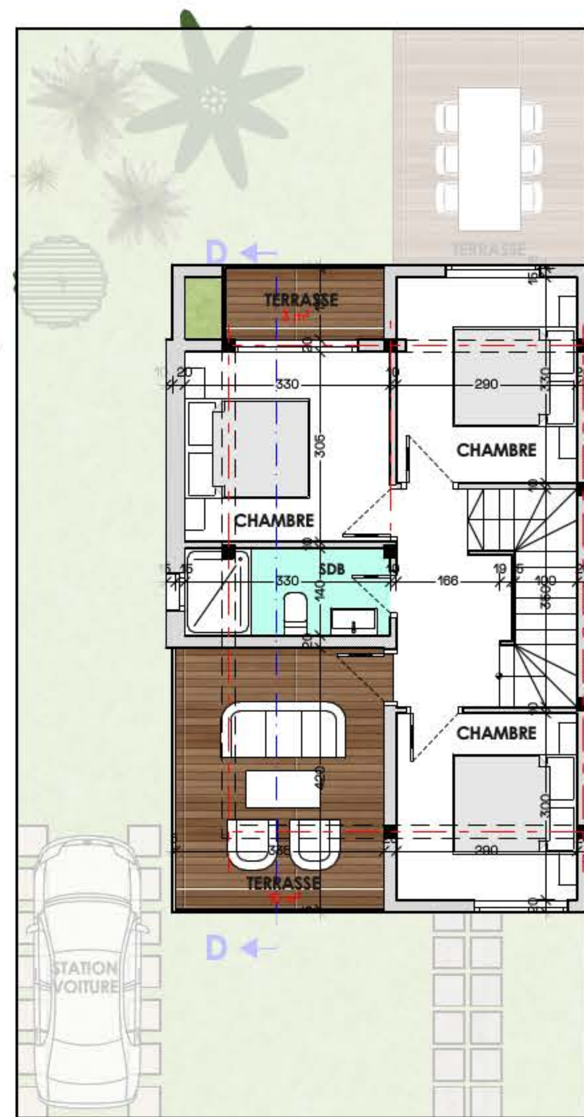
PLAN ETAGE
