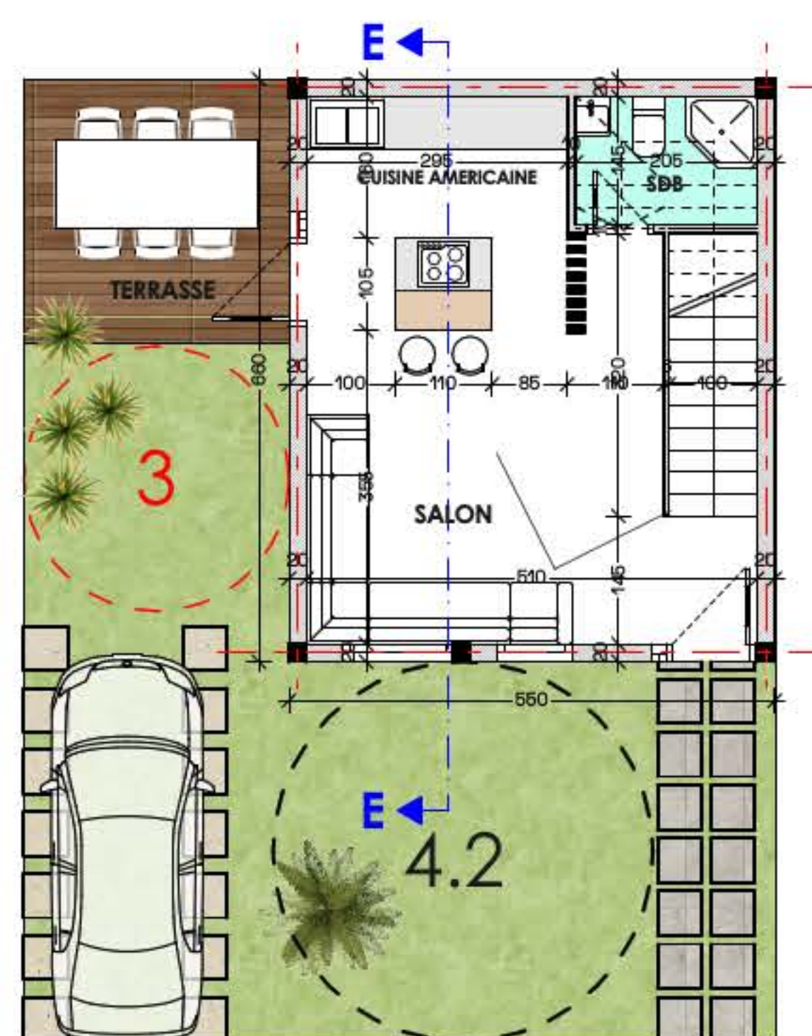
PLAN REZ-DE-CHAUSSEE
